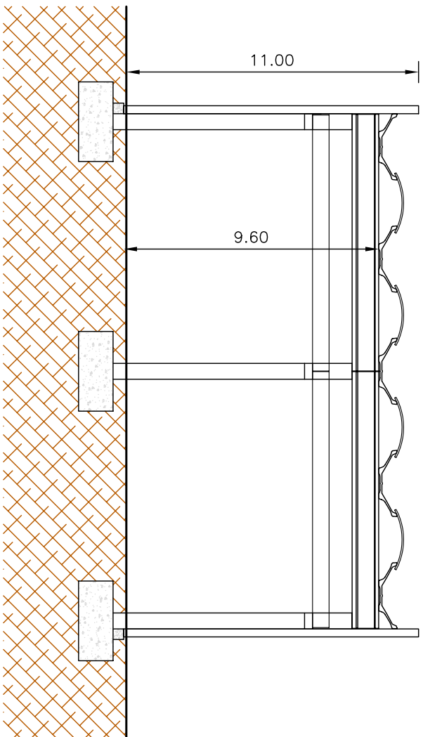
SEZIONE 1-1
