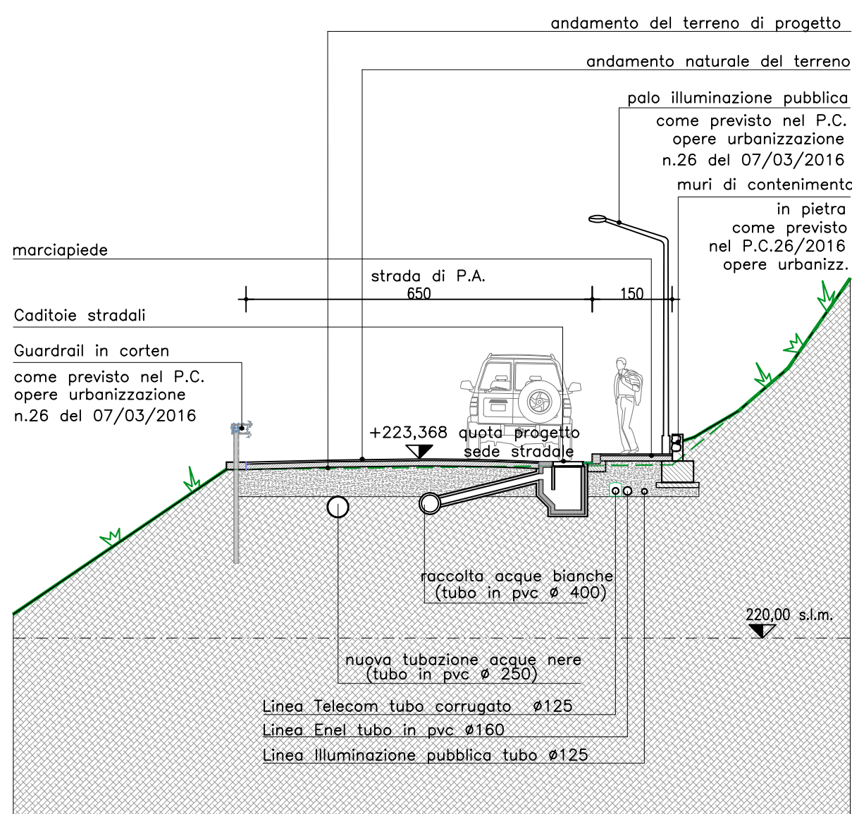
SEZIONE 1 - sezione stradale tipo scala 1:100
