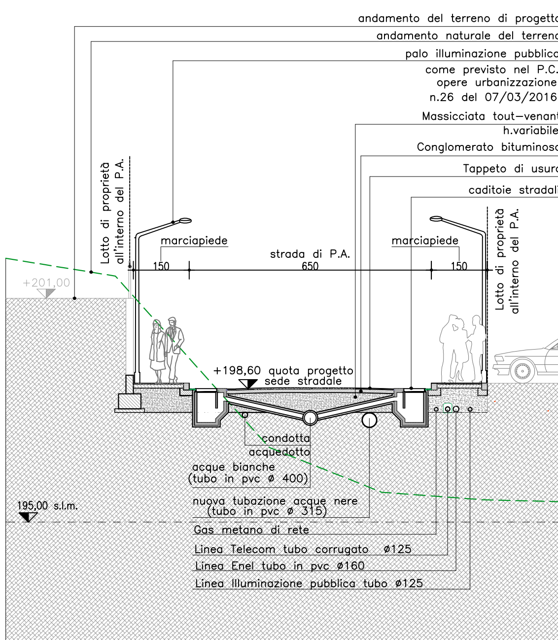
SEZIONE 2 - sezione stradale tipo scala 1:100
