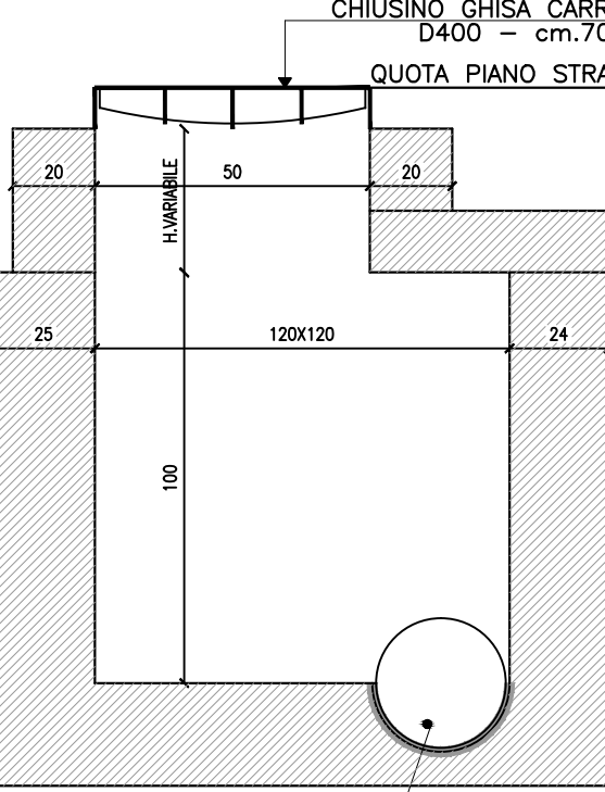
POZZETTO CON CAMERETTA D'ISPEZIONE ACQUE NERE scala 1:20
