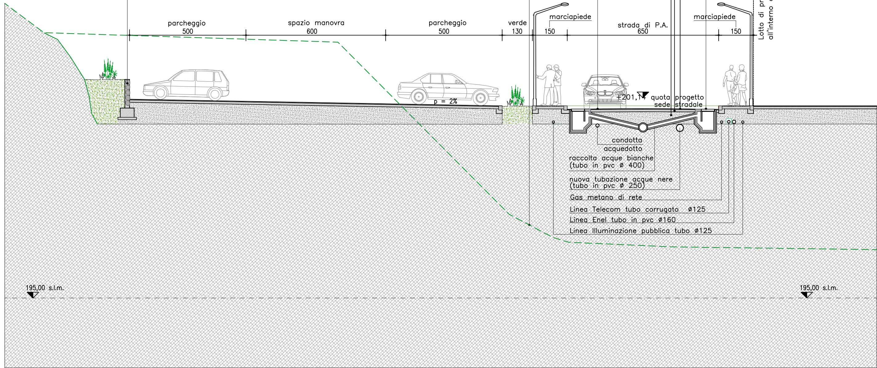
SEZIONE 1 - sezione stradale tipo scala 1:100
