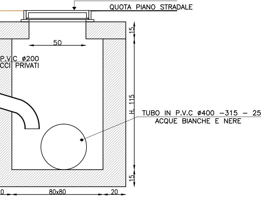
POZZETTO ISPEZIONE ACQUE BIANCHE E NERE scala 1:20
